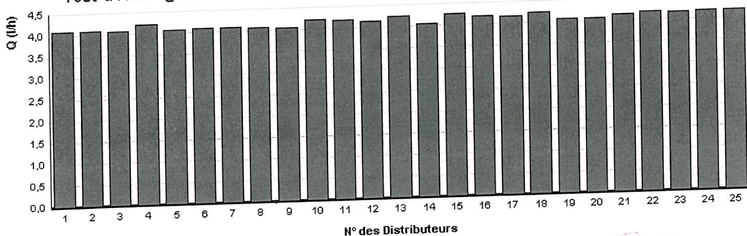
Test d'Homogénéité de fabrication du goutteur GOLD DRIP TURBULENT 4 l/h
