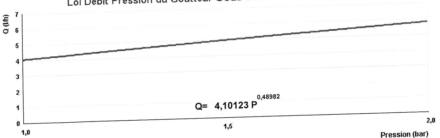
Loi Débit Pression du Goutteur GOLD DRIP TURBULENT 4,00 l/h
