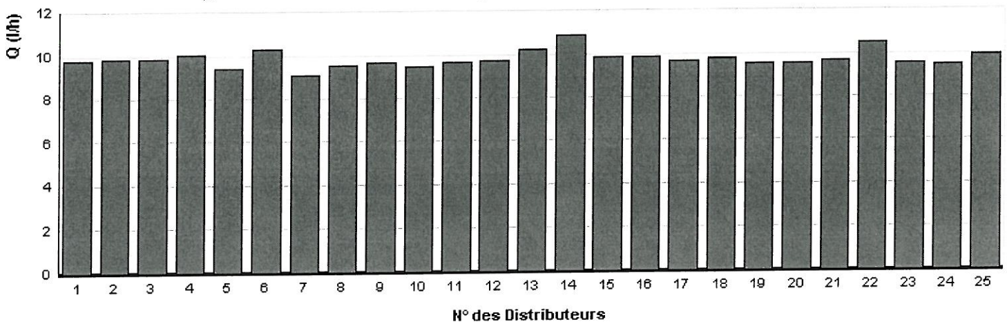
Test d'Homogénéité de fabrication du goutteur MBTECH AUTOREGULANT 8,5 l/h
