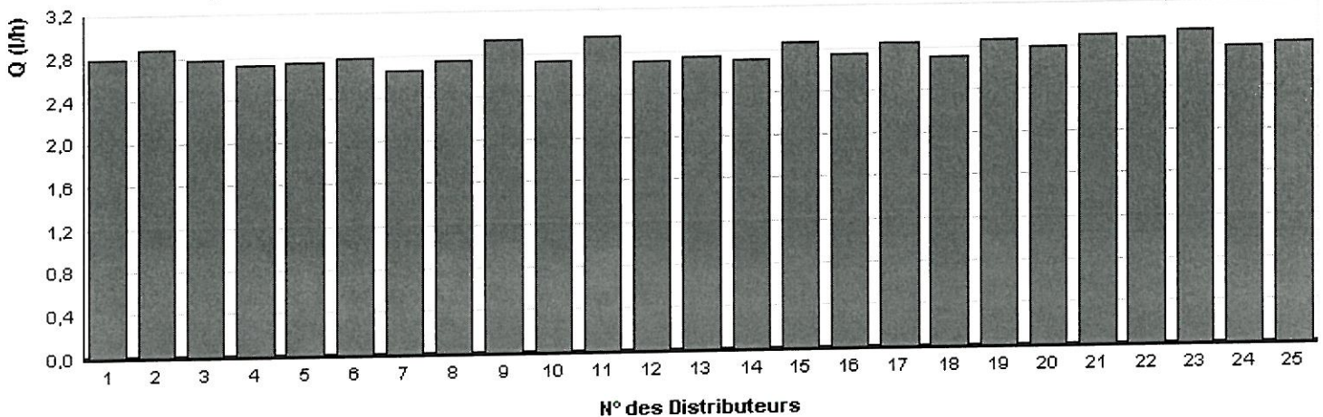
Test d'Homogénéité de fabrication du goutteur AZUD PREMIER PC AUTOREGULANT 3 l/h
